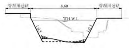
河道改修区間(省路橋上流)横断面図
