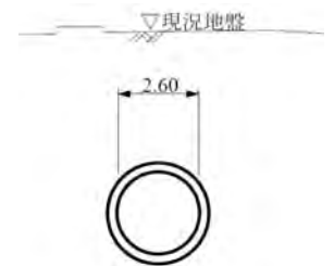
パイパス水路区間横断面図
