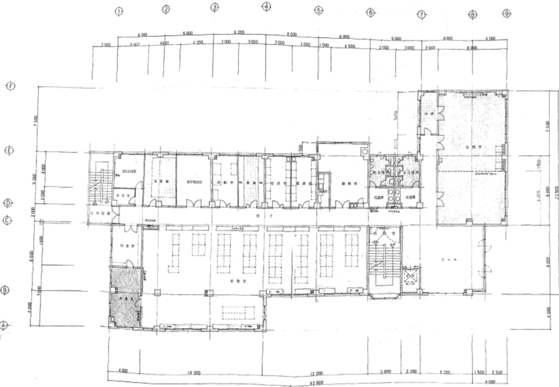
2階平面図
