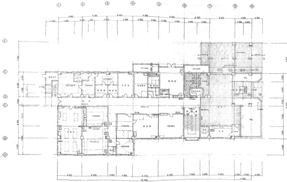
1階平面図
