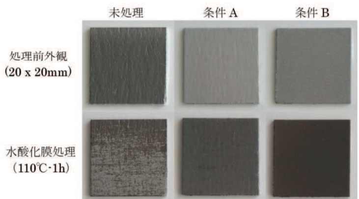
(1)水酸化膜処理前後の試験片外観
