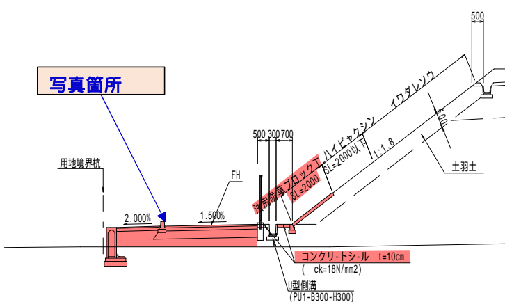
施工横断図（側道）
