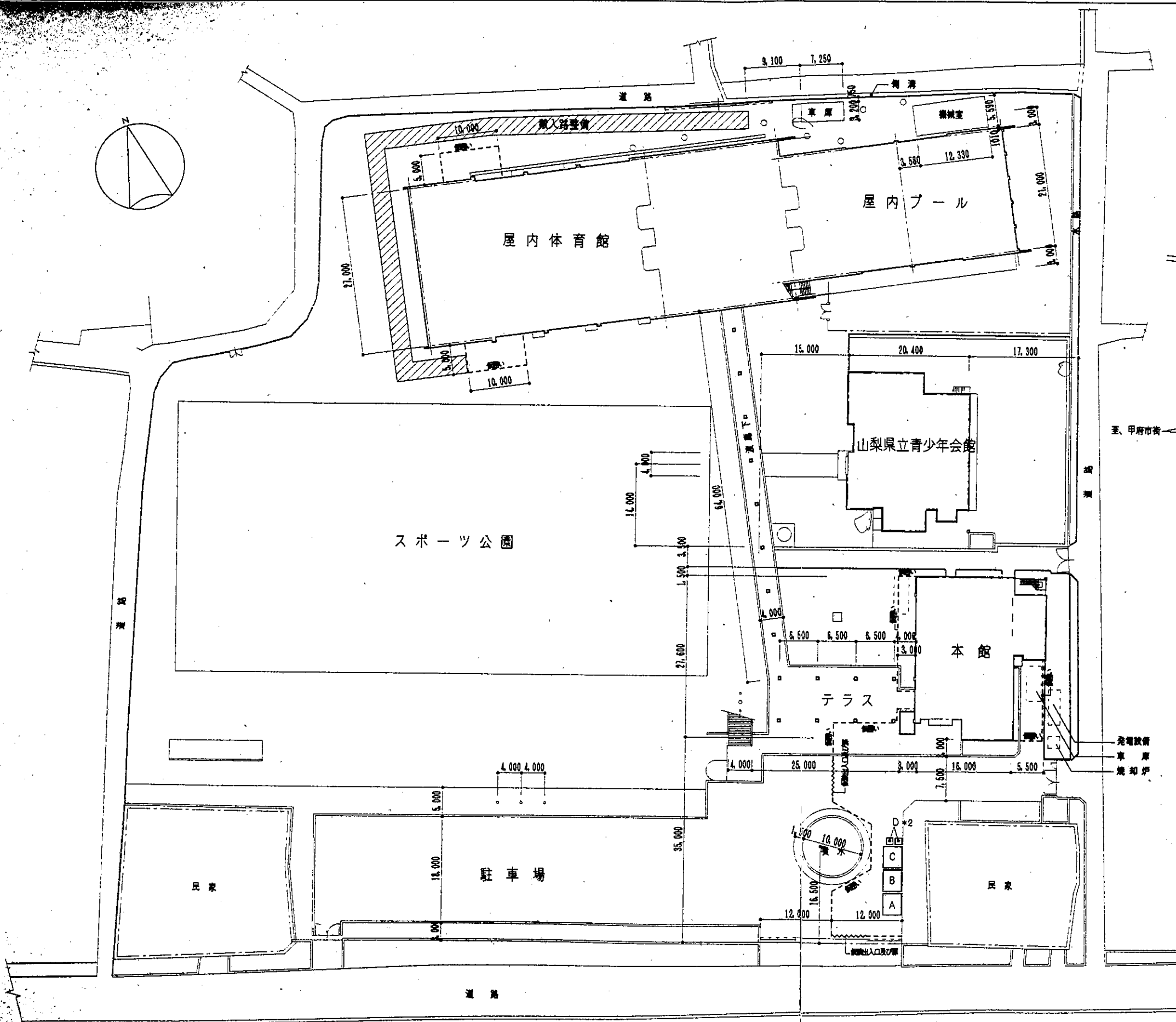
配置図 S=1/500
