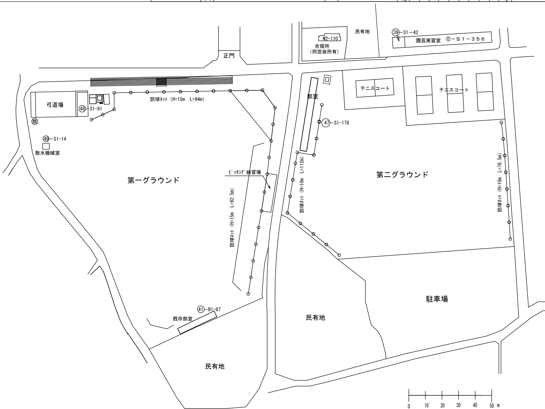
配置図 2
