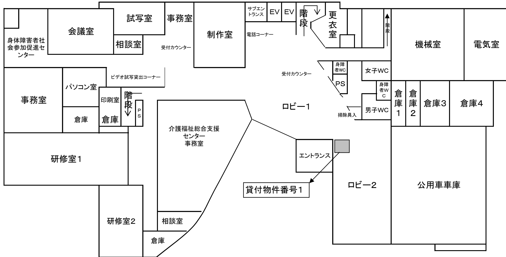
位置図（貸付物件番号1） 山梨県福祉プラザ 平面図(1階)
