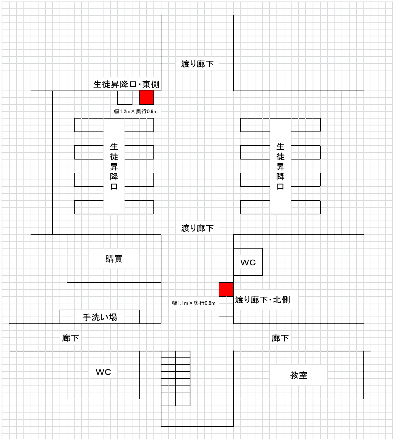
山梨高校生徒昇降口及び渡り廊下見取図
