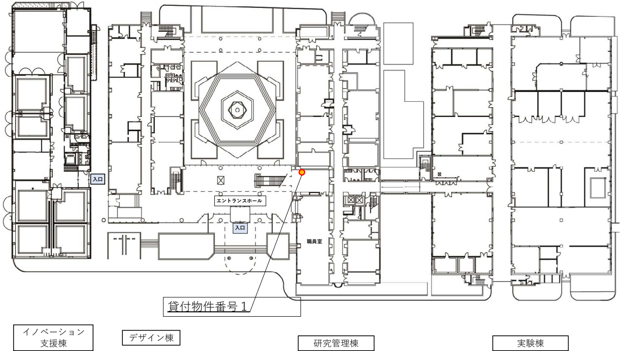
産業技術センター 1階配置図 (イノベーション支援棟、デザイン棟、研究管理棟、実験棟)
