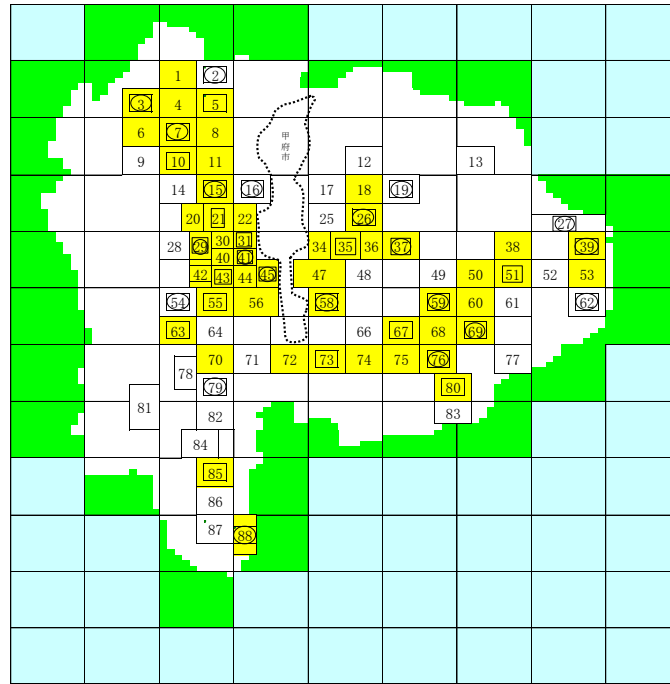
令和3年度地下水測定地点図(環境基準項目・要監視項目)
