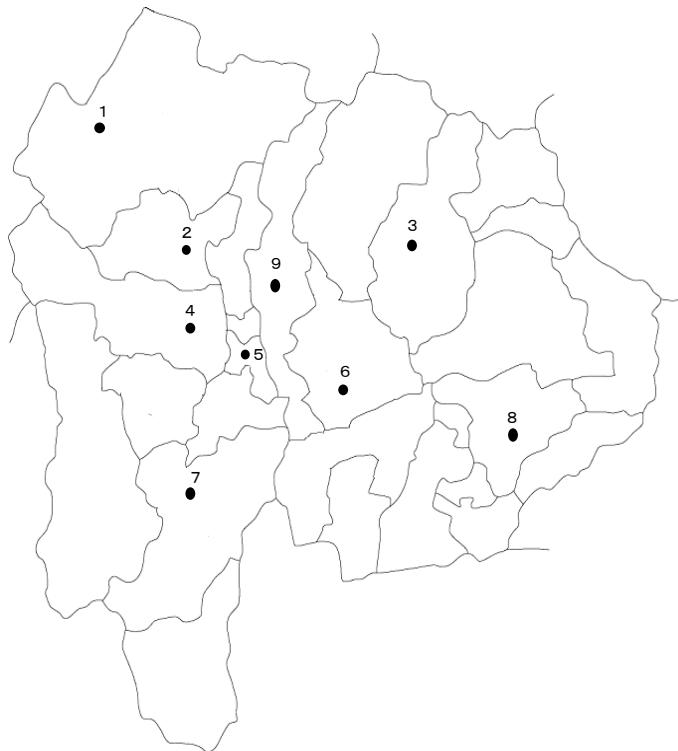
令和3年度ダイオキシン類常時監視地点図 地下水
