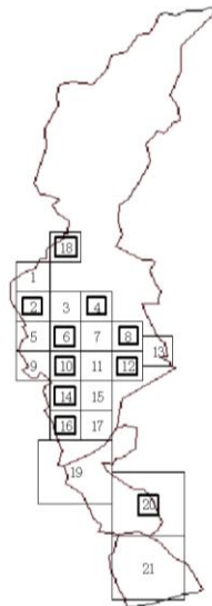
令和32年度地下水測定地点図(環境基準項目・要監視項目)
