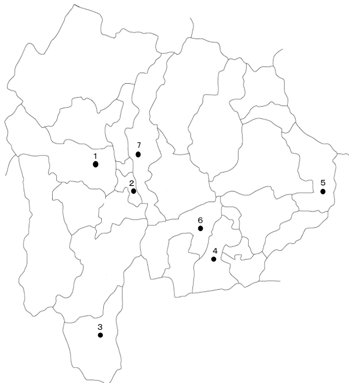
令和3年度ダイオキシン類常時監視地点図 土壌
