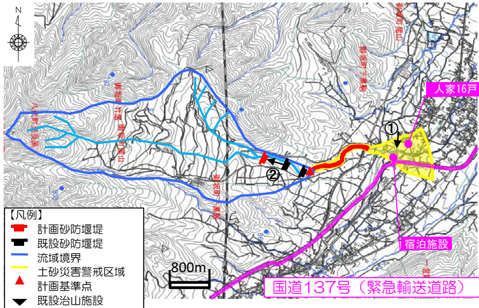
【流域概要図】
