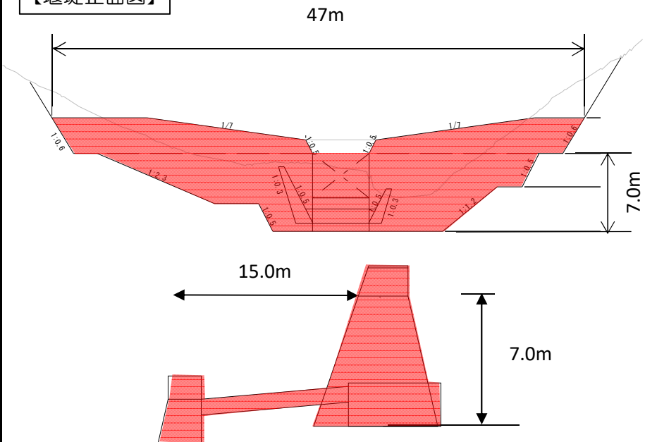
【堰堤正面図】
