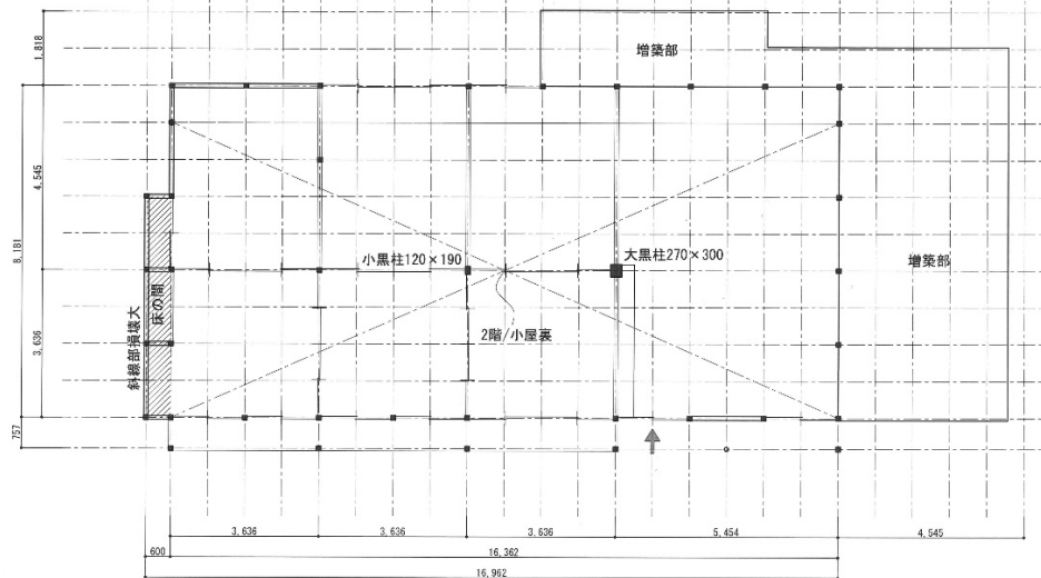
間取図2階
