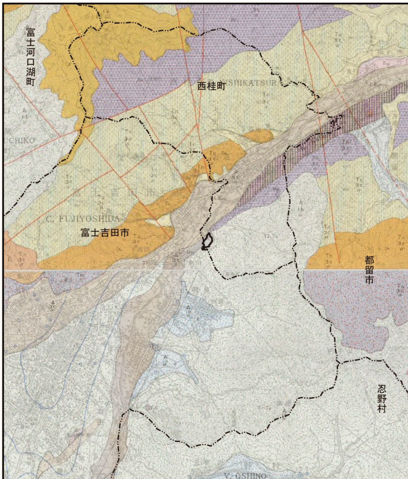
図2.1-13(1) 表層地質図
