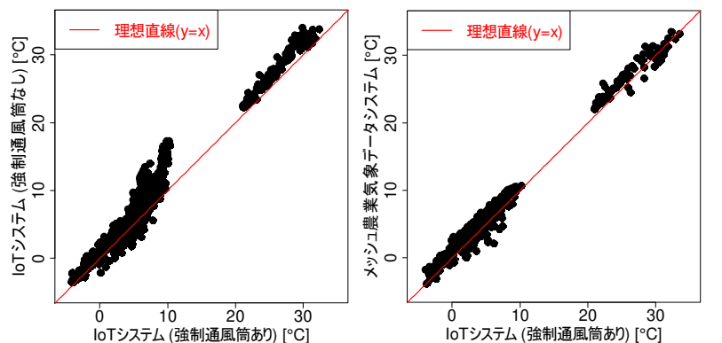
(a) 強制通風筒のないIoTシステム (b) メッシュ農業気象データシステム 図1 強制通風筒搭載IoTシステムとの温度の相関
