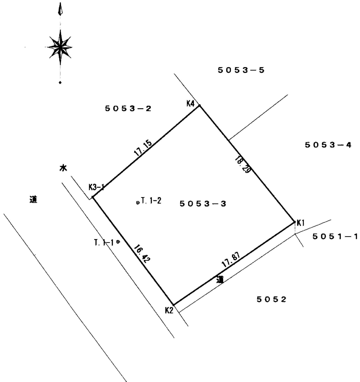
座標面積計算表（任意座標）
