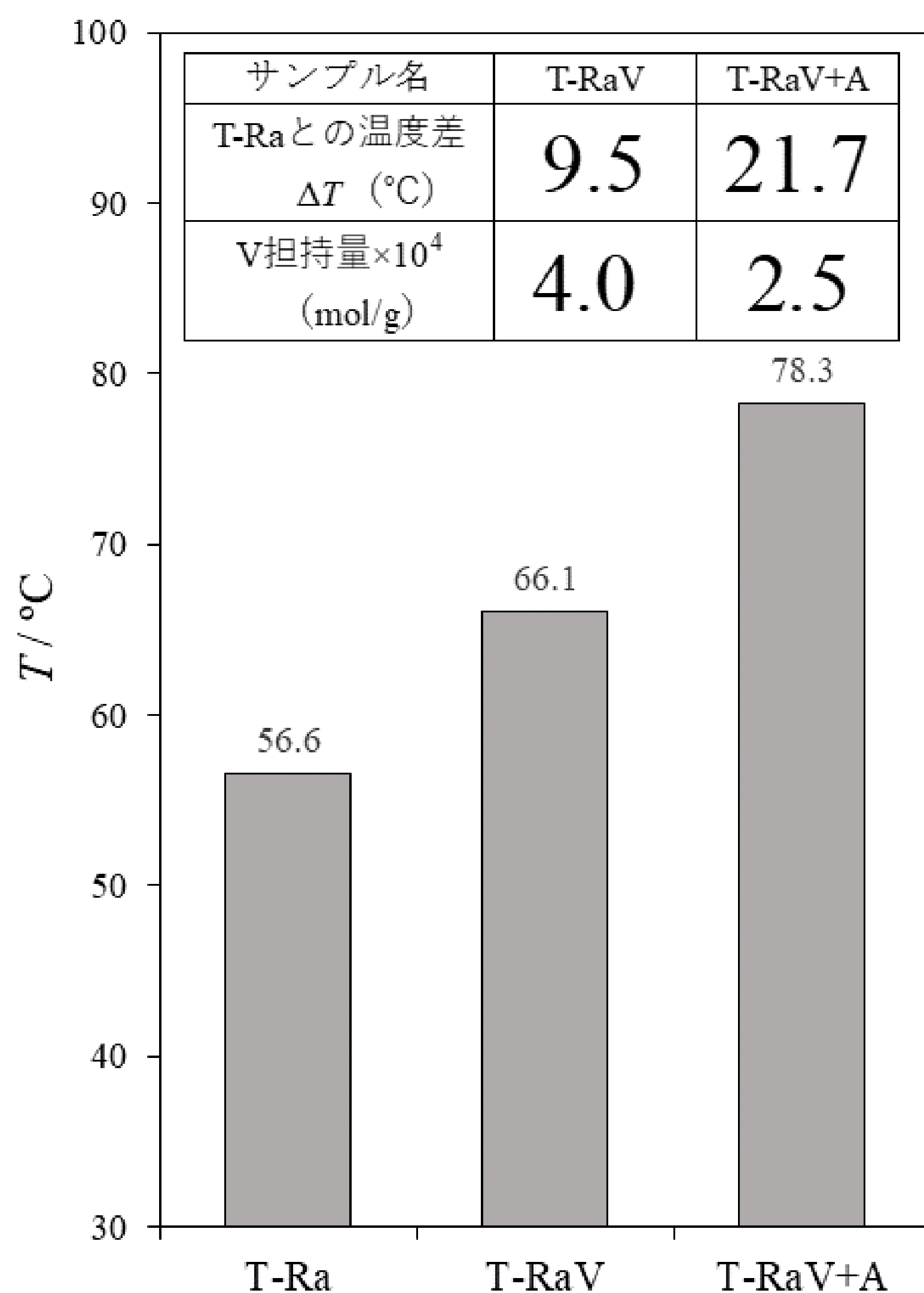
図2 光吸収発熱性の評価
