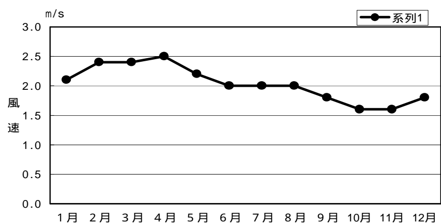
図 - 1 - 1 . 1 気象の状況 ( 甲府地方気象台 ) ( 1985 ~ 2004年の平均値 )
