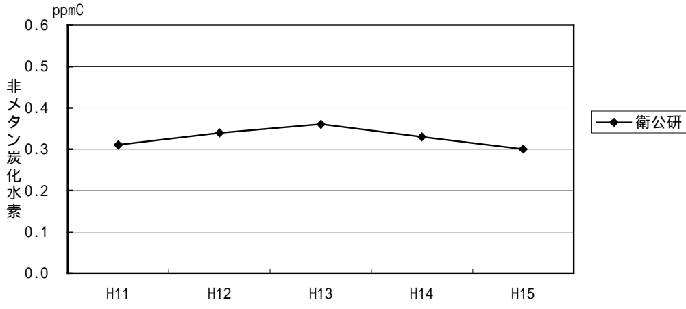
図 - 2 - 7 . 2 大気汚染濃度の経年変化(平成11年~15年度)
