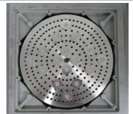
図3 装置の概要と最適条件の磁石配置
