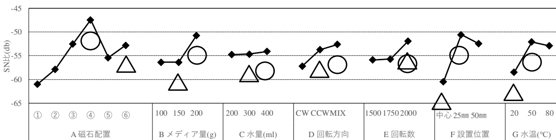
図2 要因効果図(○:最適条件 △:現行条件)
