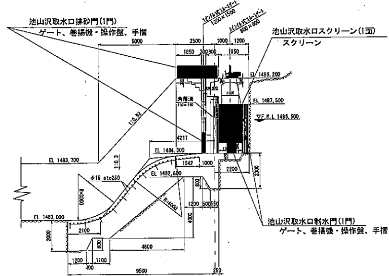
断面図(池山沢取水口)
