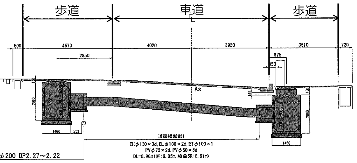
標準横断図
