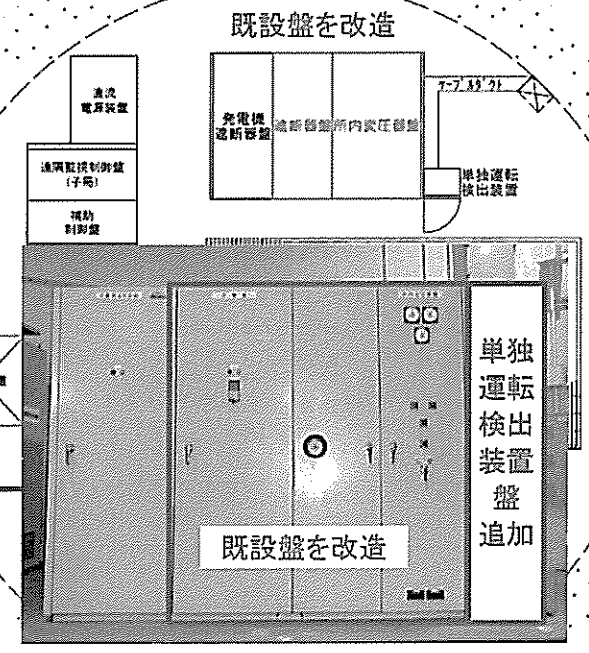
藤木発電所内 機器配置図(更新後)
