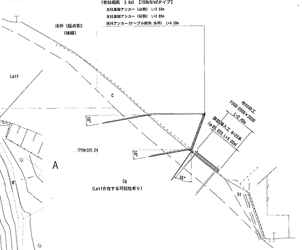
標準横断図(A-A)
