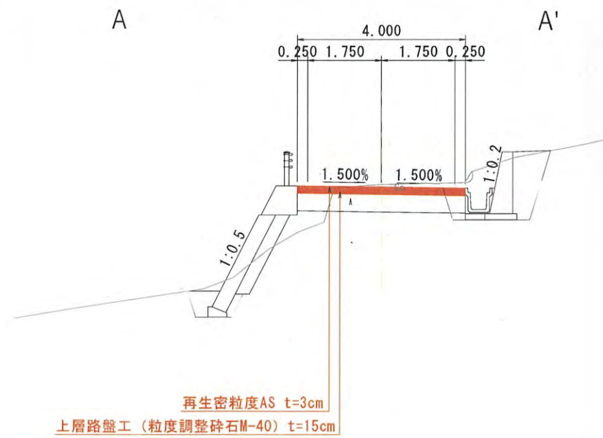
標準断面図
