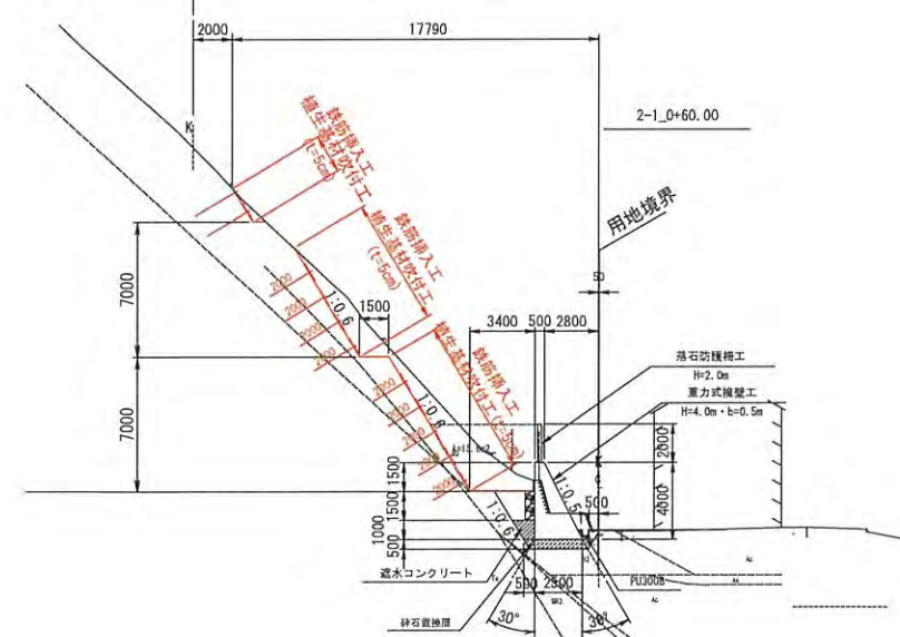
標準横断図
