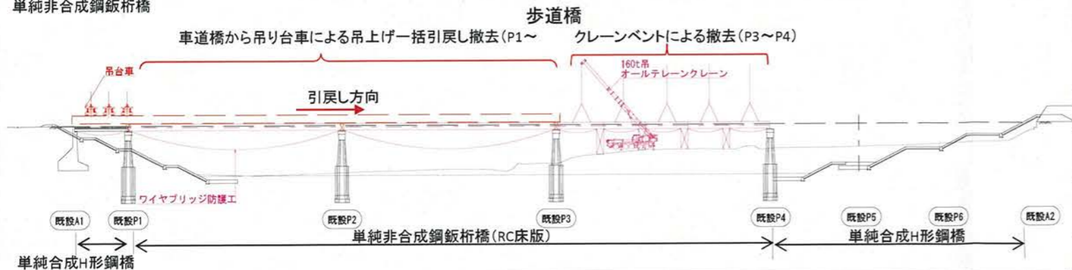
撤去図
