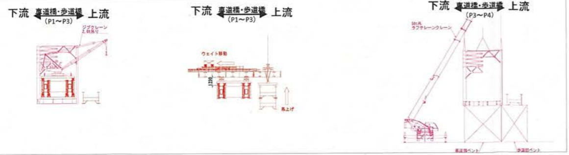
撤去図
