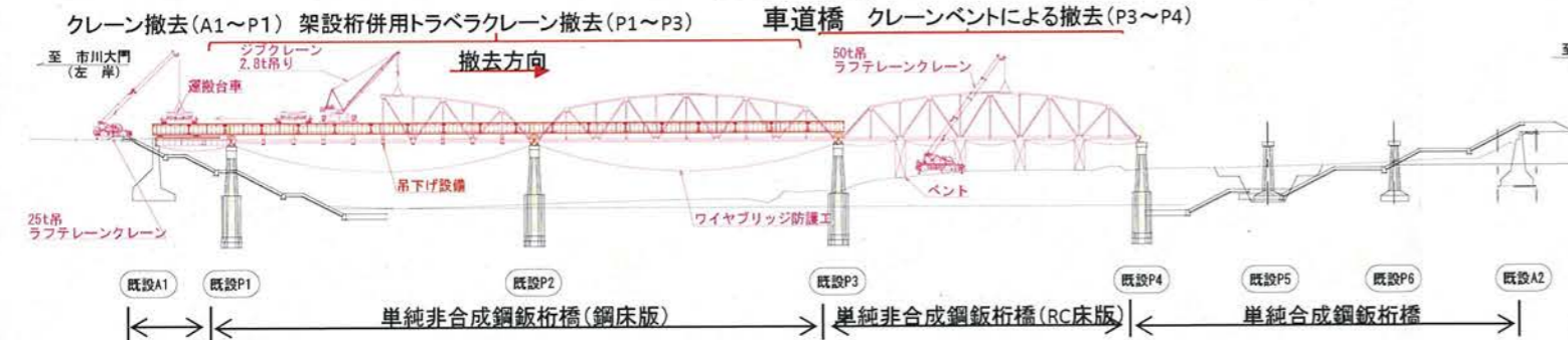
側面図
