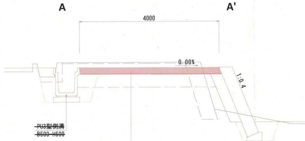
標準断面図
