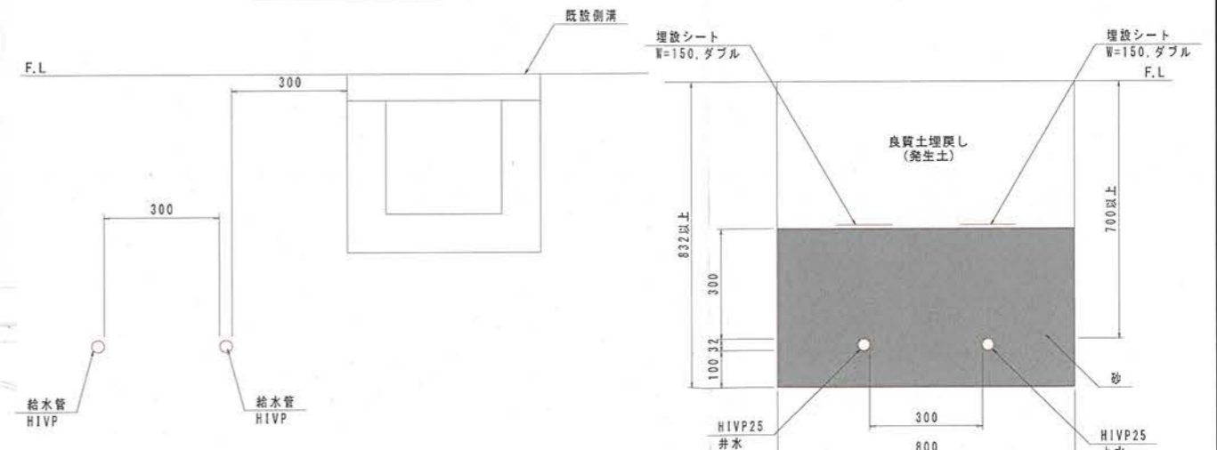
配水管
