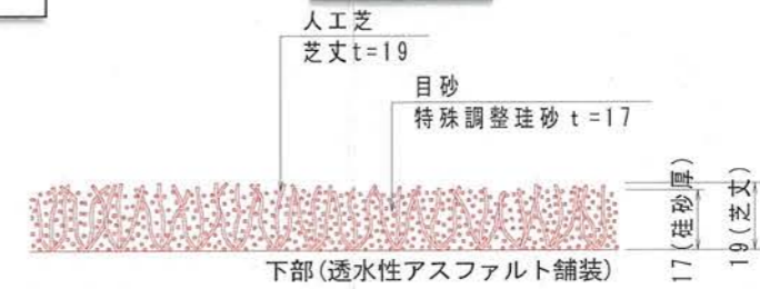
詳細図
