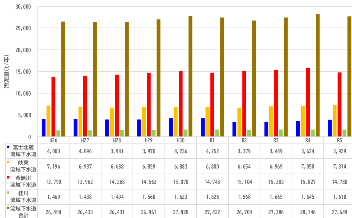
【図5-2 流域下水道から発生する汚泥量の推移】
