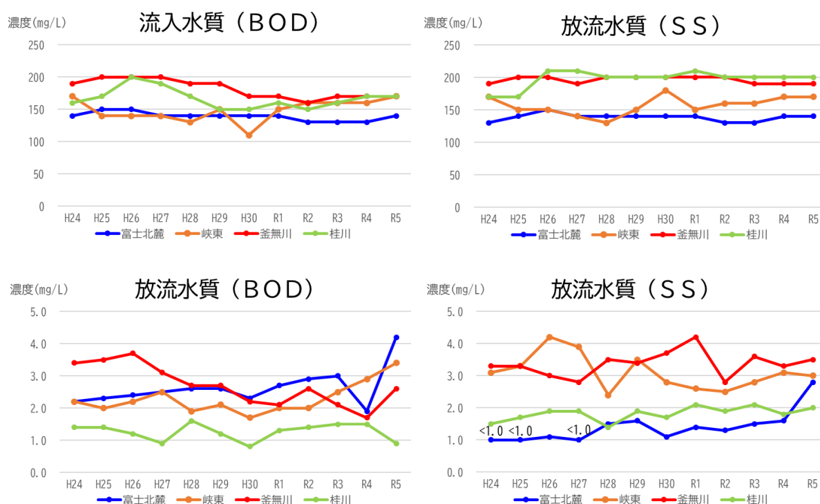
【図5-1 流入水質及び放流水質の経年変化（年平均値）】
