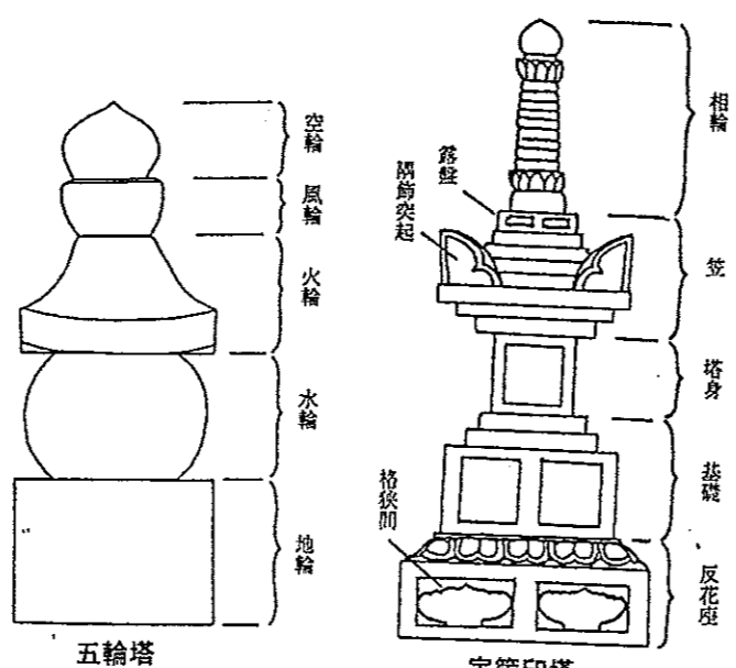
図12 五輪塔・宝篋印塔の部分名称
