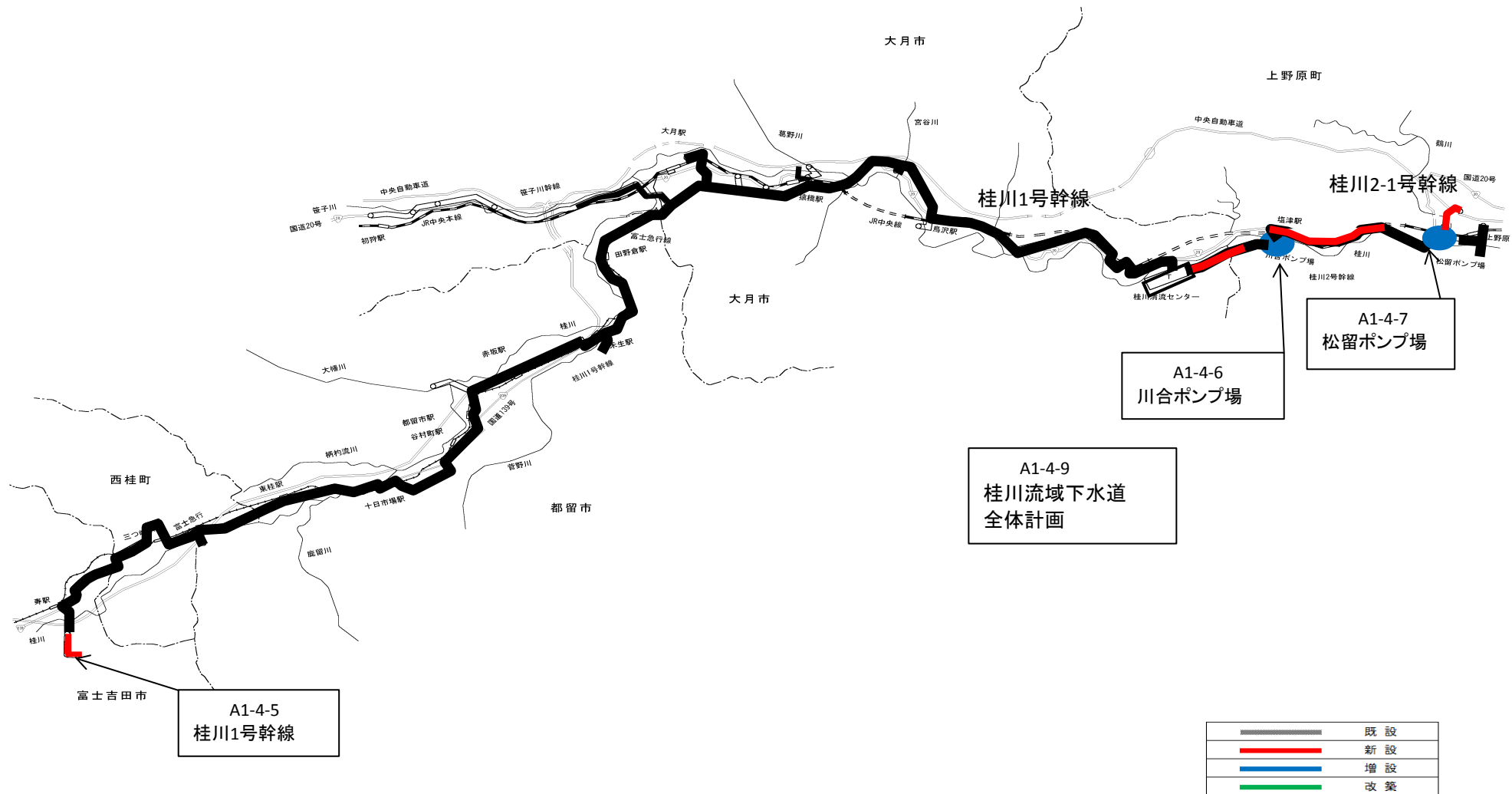
桂川流域下水道計画図
