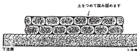
控え土のう正面図
