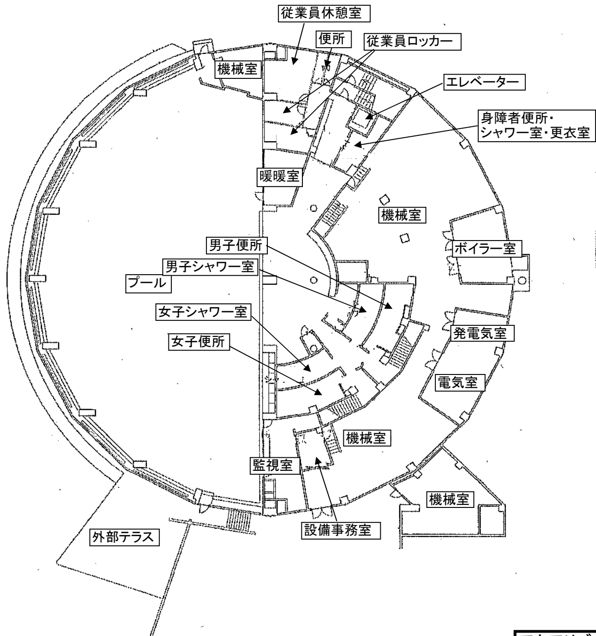
アクアリゾート清里平面図(1F)
