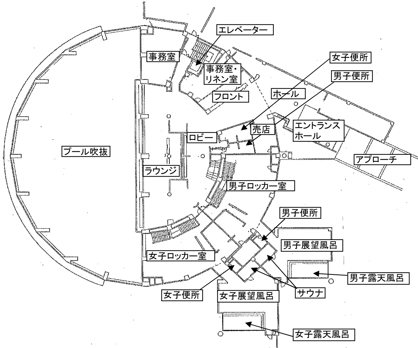
アクアリゾート清里平面図(2F)
