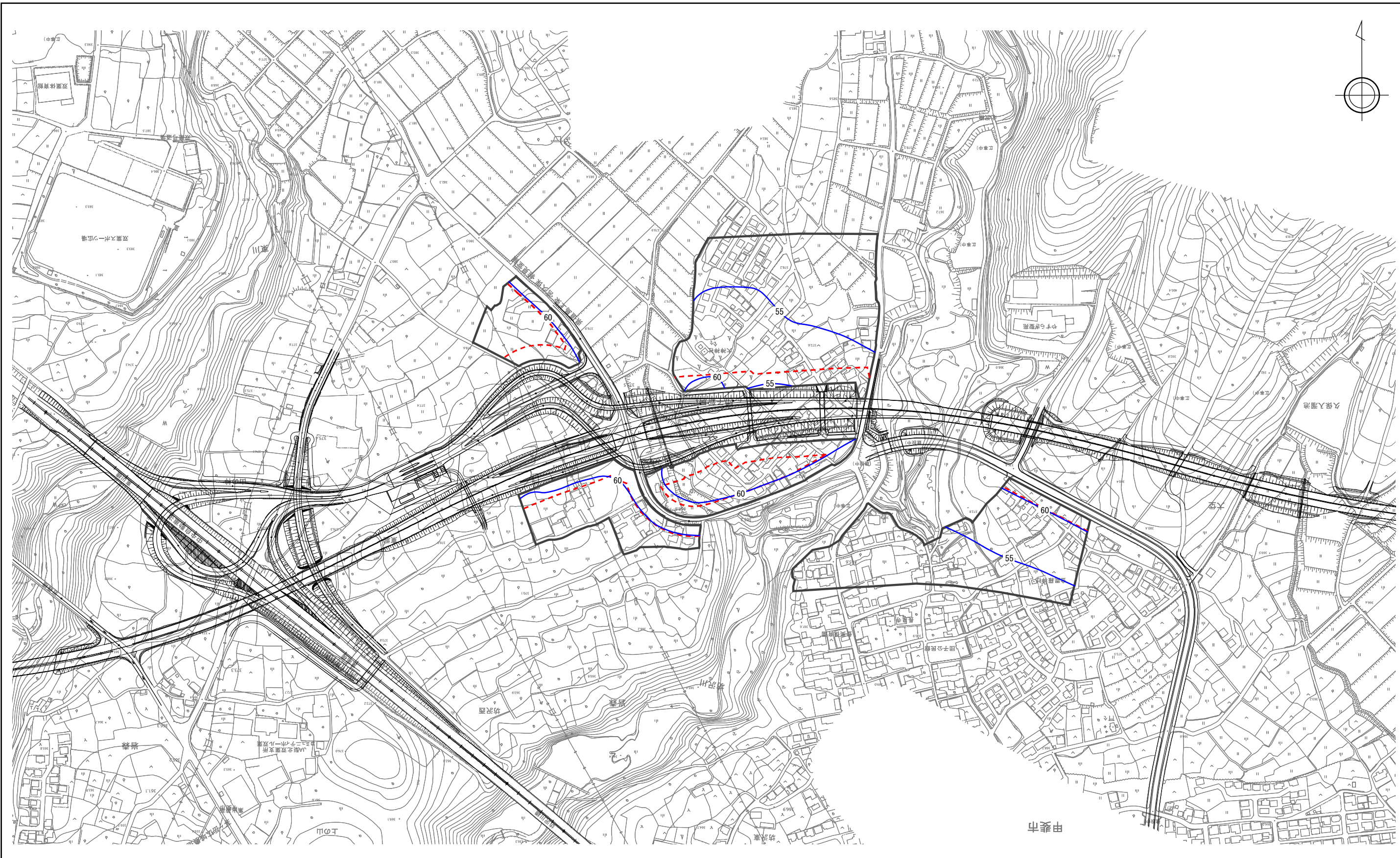
図 4-4-1 (4) 等音分布図 (甲斐 IC・JCT 周辺 夜間 4.2m)
