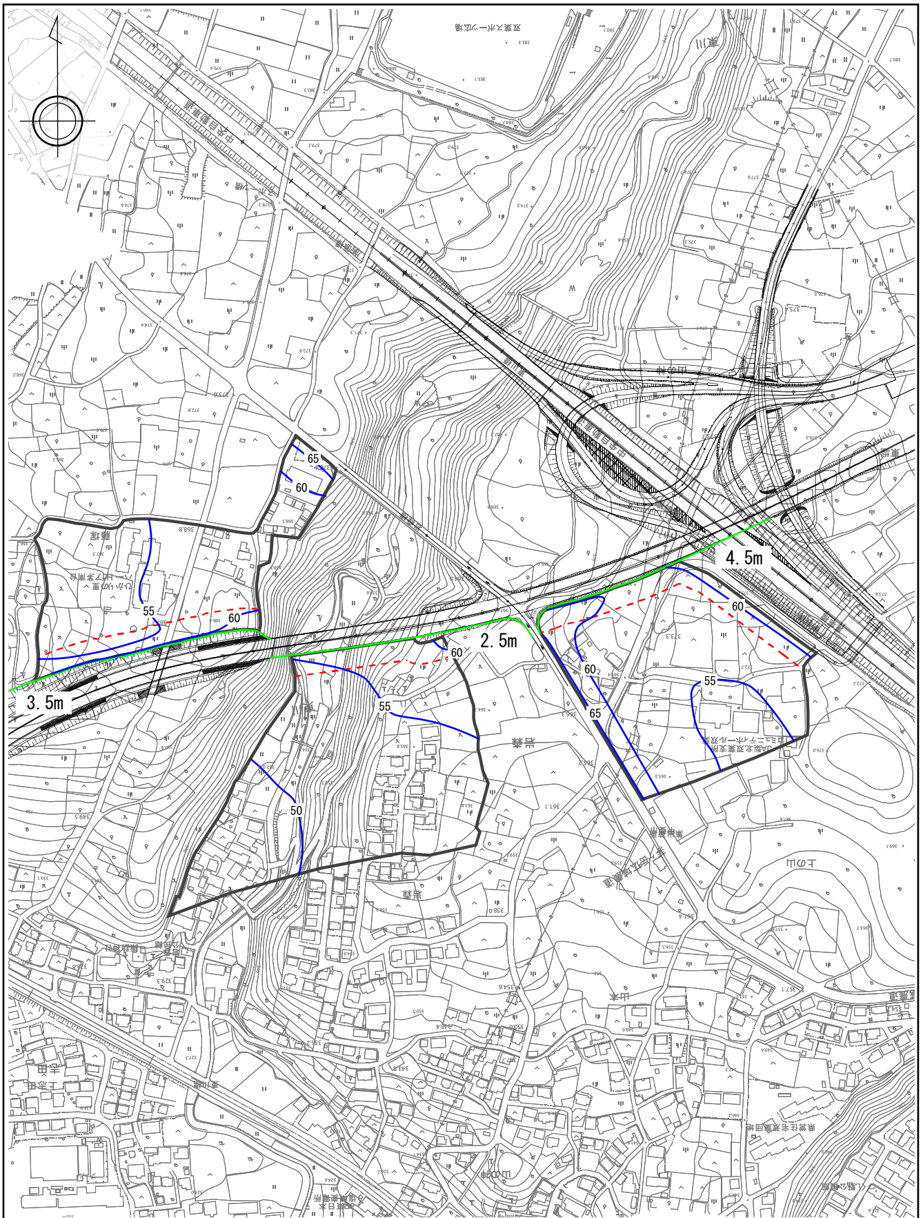
図 4-5-1 (4) 等音分布図 (岩森交差点周辺 夜間 4.2m)
