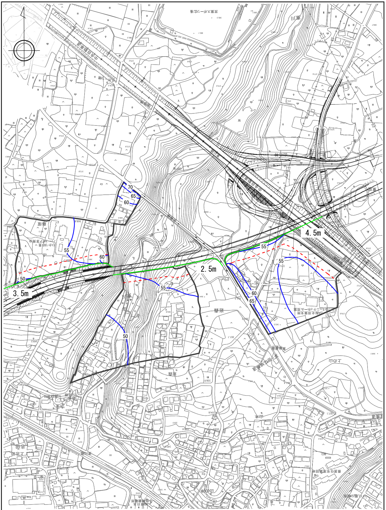
図 4-5-1 (3) 等音分布図 (岩森交差点周辺 夜間 1.2m)
