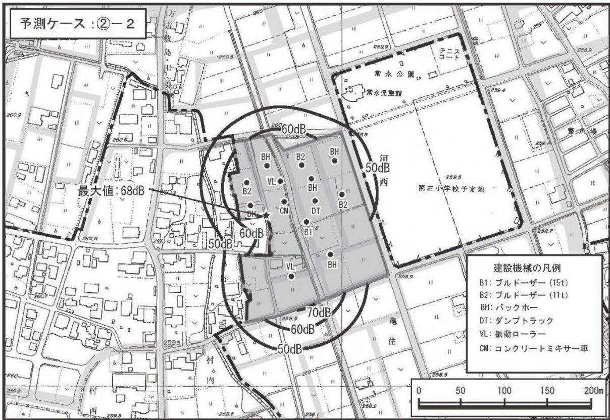
図 2 - 1 - 2 (b) 平成 2 1 年度 事後調査 振動調査候補地点
