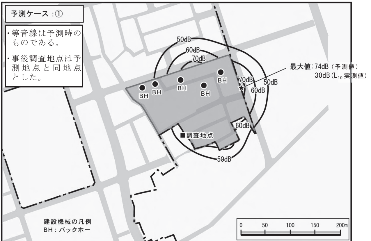
図 2 - 1 - 4 (a) 平成 20 年度 事後調査 振動調査地点及び建設機械の稼動状況
