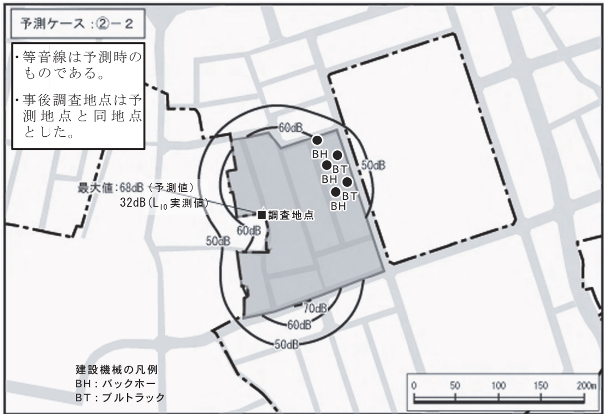
図 2 - 1 - 4 (b) 平成 2 1 年度 事後調査 振動調査地点及び建設機械の稼動状況
