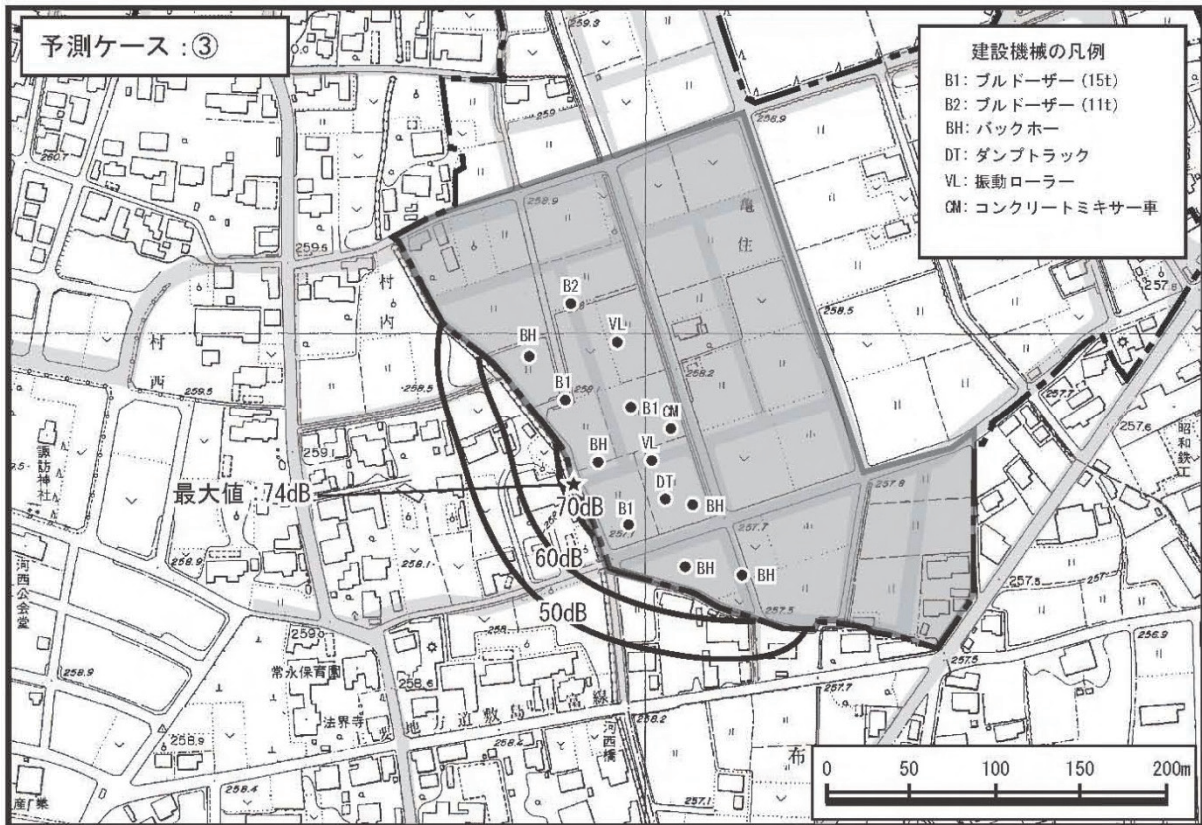
図 2 - 1 - 2 (c) 平成 2 2 年度 事後調査 振動調査計画地点
