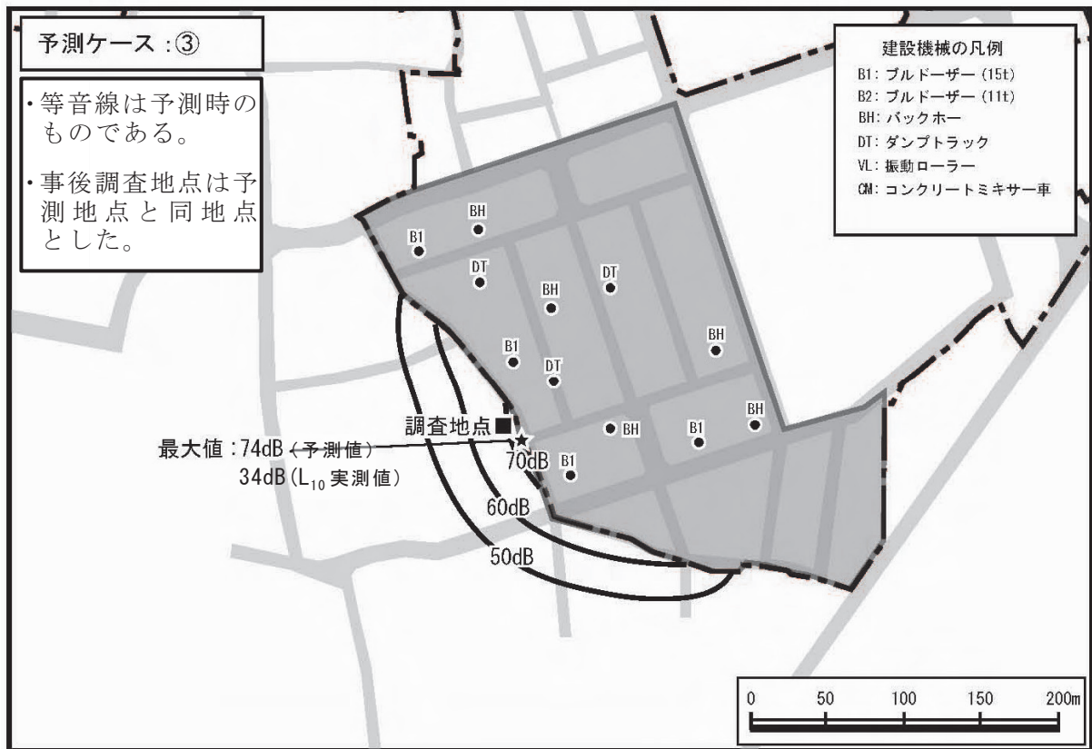
図 2 - 1 - 4 (C) 平成 2 2 年度 事後調査 振動調査地点及び建設機械の稼動状況
