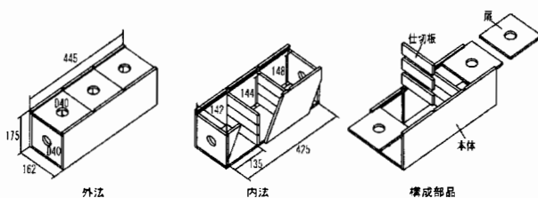
Fig. 2 ワインケースの形状と構成部品
