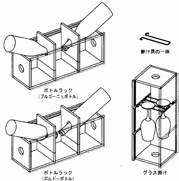
Fig. 3 ボトルラックとグラス掛け
