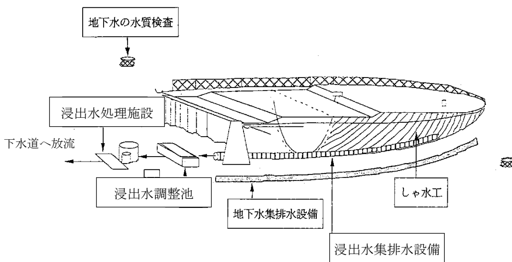
図 2-2-9 最終処分場のイメージ図
