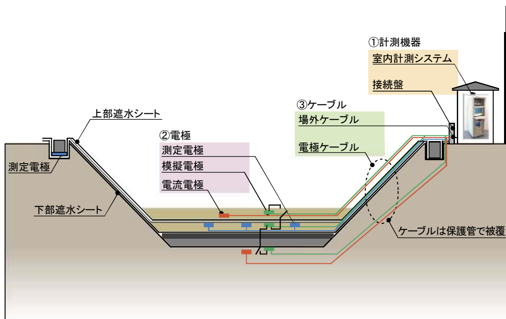
図 2-2-10 点電極・電位比抵抗方式(漏洩電流式)電気検知システム設備断面図(A—A 断面)
