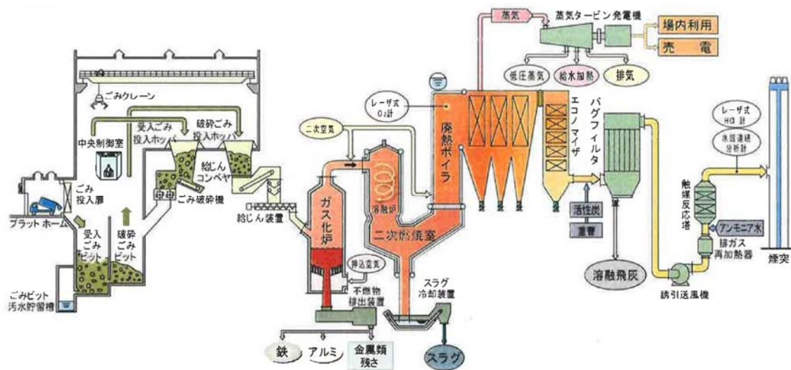
図 2-2-5 焼却溶融施設の処理フロー(ガス化溶融)
