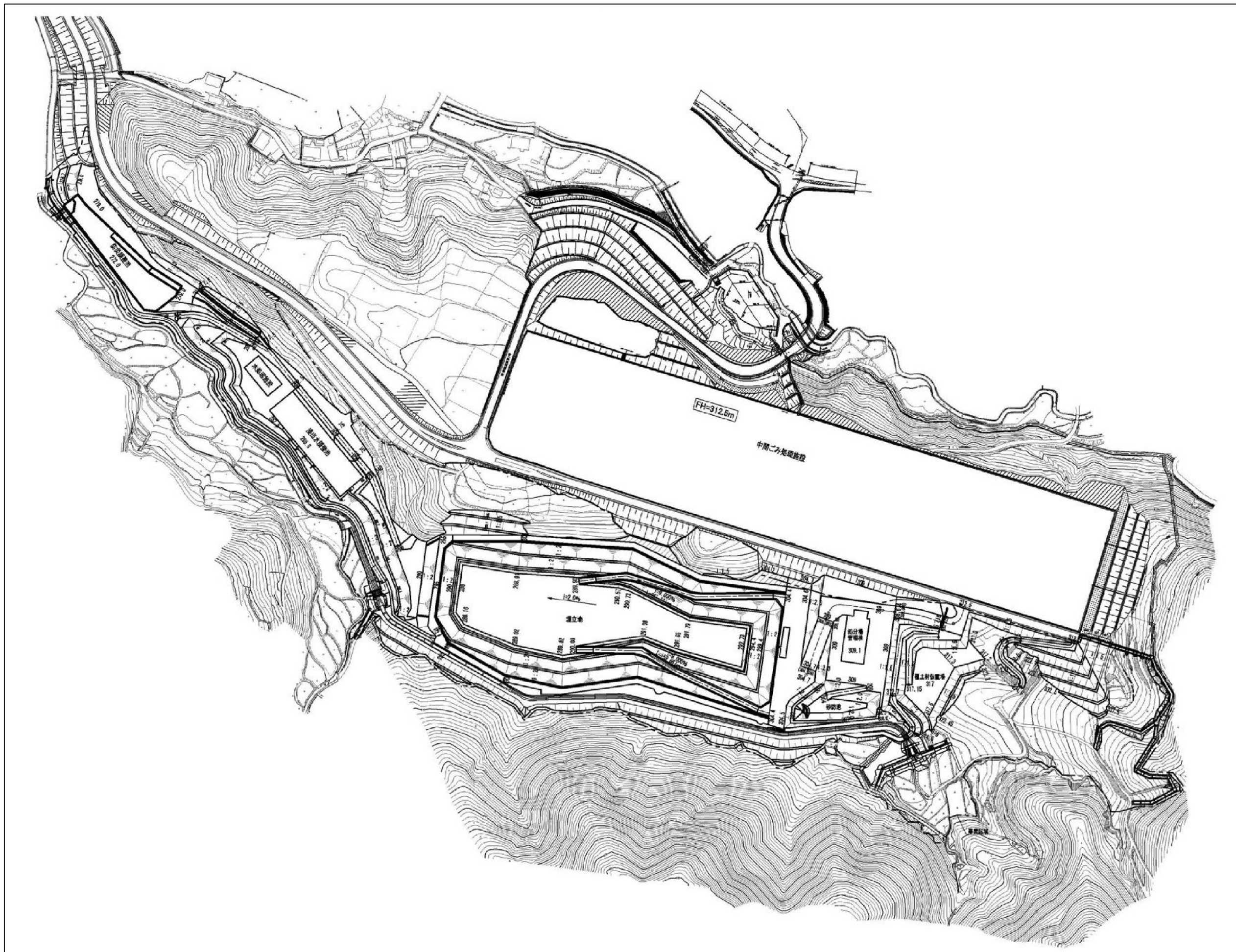
図 2-2-7 最終処分場平面計画図
