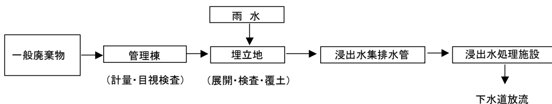
図 2-2-13(2) 最終処分場の処理フロー
