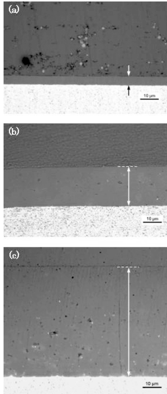
図 1 陽極酸化処理を行った試験片の断面観察写真 (処理時間:(a) 5 min,(b) 30 min,(c) 120 min)
