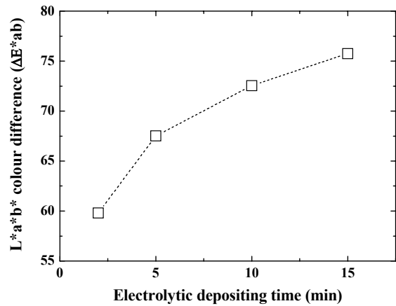
図4 電解析出時間に伴う色差変化
