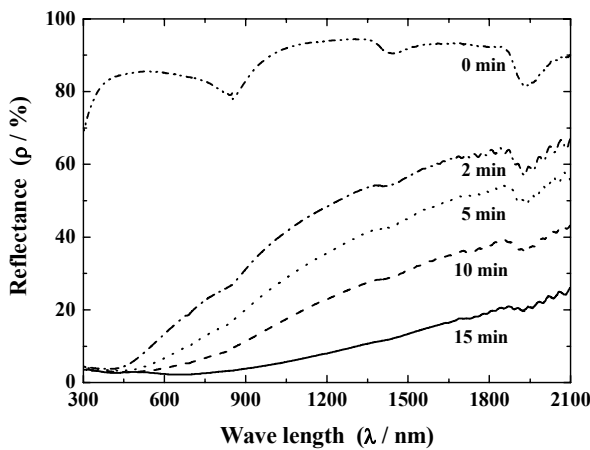
図 5 電解析出時間に伴う分光反射率 \rho の変化
