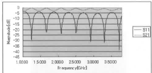
図6 反射係数 (S11) 及び伝送利得 (S21) 実測値
