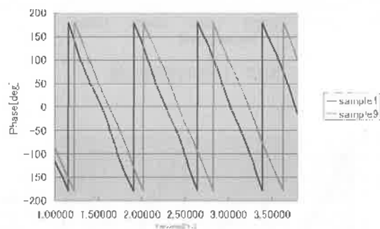
図21 位相特性測定値
