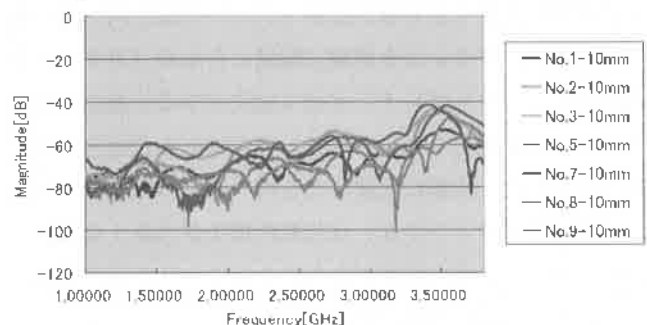
図24 近傍磁界測定値（基板-プローブ間距離10mm）
