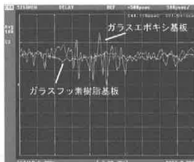
図12 群遅延時間測定値 ガラスエポキシ基板とガラスフッ素樹脂基板の比較
