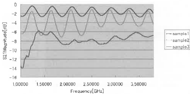
図14 伝送利得測定値
