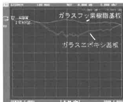
図11 伝送利得(S21)測定値 ガラスエポキシ基板とガラスフッ素樹脂基板の比較
