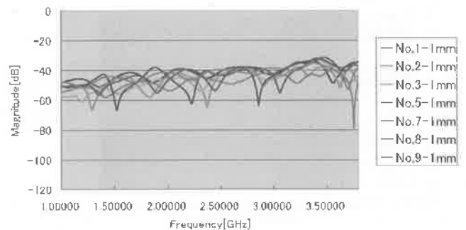
図22 近傍磁界測定値（基板-プローブ間距離1mm）
