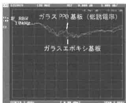
図10 伝送利得(S21)測定値 ガラスエポキシ基板とガラスPPO基板(低 \epsilon )の比較
