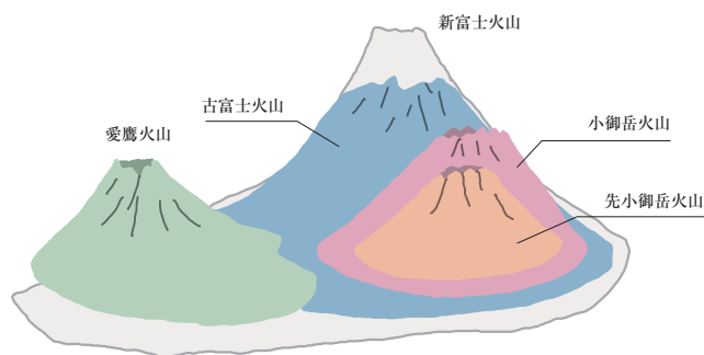
富士山の構造(富士山の下に埋まる古い火山体)
