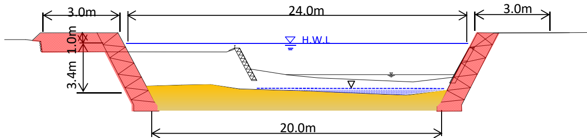
標準横断面図(イメージ)
