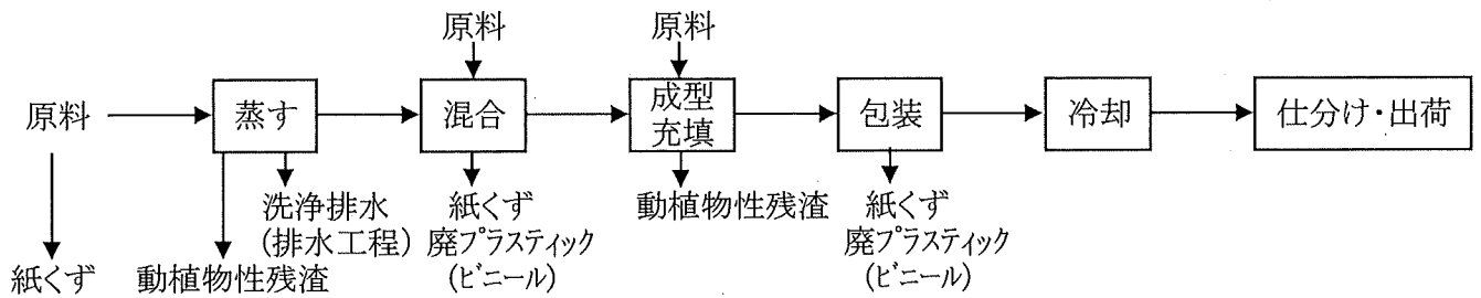
図 3 和菓子製造フローシート
