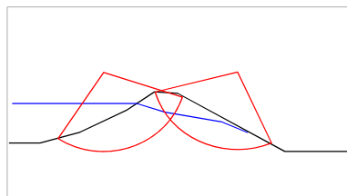
ため池堤体の安定性を解析
