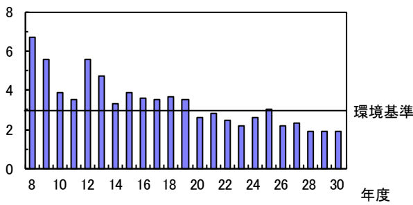
BOD 75%値(mg/L)
