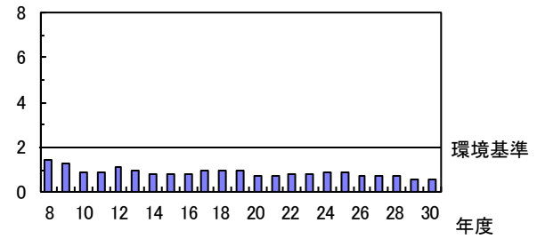
BOD 75%値(mg/L)
