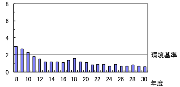
BOD 75%値(mg/L)
