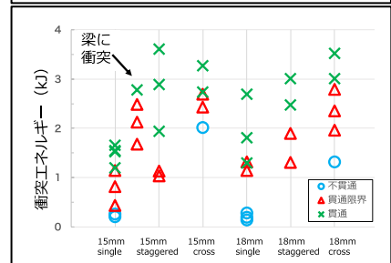
図2 クロス構造とスタッカー構造の衝突エネルギーの実験結果
