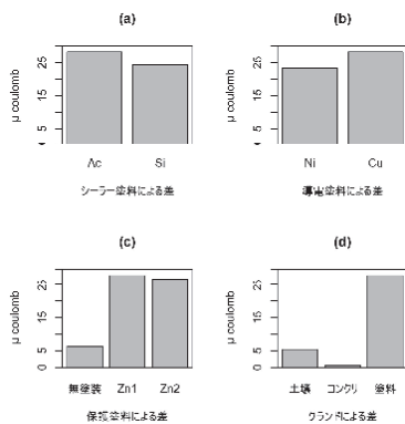
図1 コンクリートに塗布した下地、導電、保護面の塗料種類別導電性。Ac, Siはアクリル系、シリコン系下地塗料、Ni, Cuはニッケル系、銅系塗料。Zn1, Zn2は亜鉛防錆塗料1、亜鉛防錆塗料2の略称。(d)は電気柵の電極を土壌、無塗装コンクリート、塗装コンクリートに接触させた時の導電性を示す。
