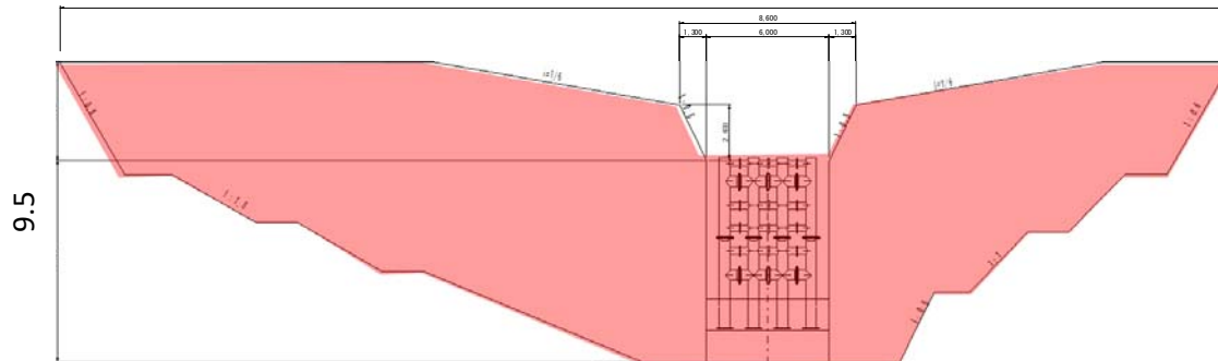
堰堤正面図
